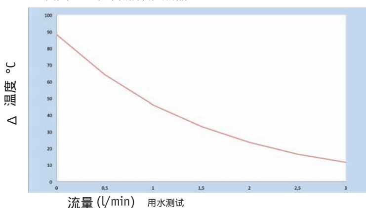
温度图 - 物料流体加热器
