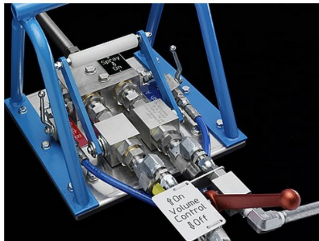
Mischblock
