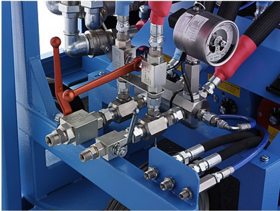
Anschlussblock für das Schlauchpaket
