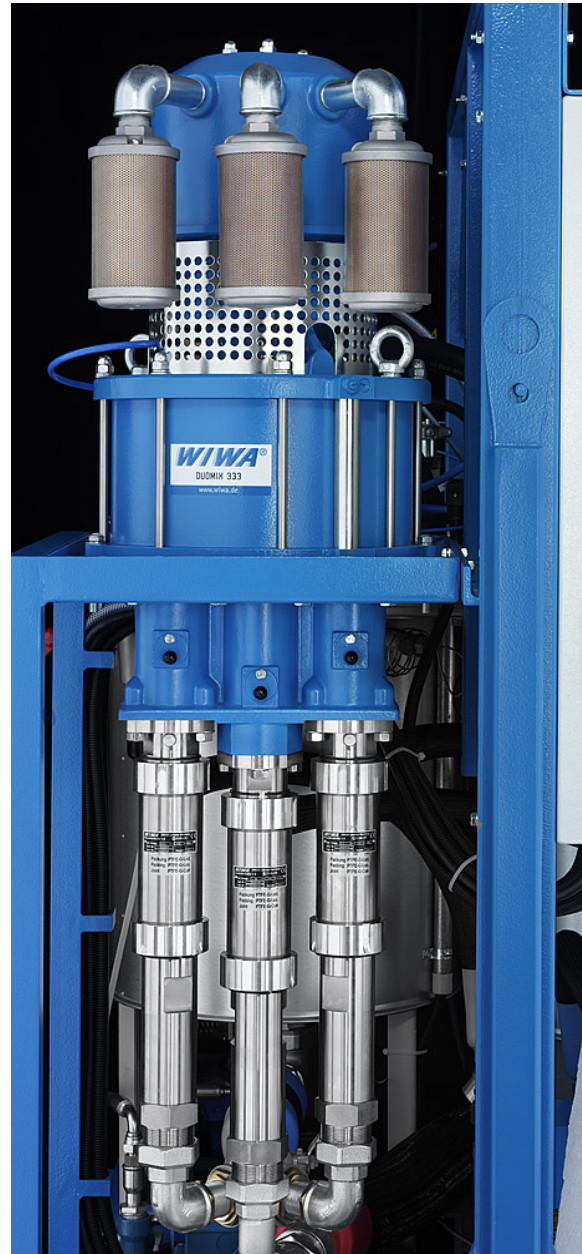
主泵（含空气马达和物料泵）
