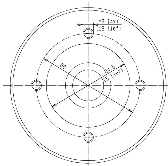
Ansicht A (Pos.44)
